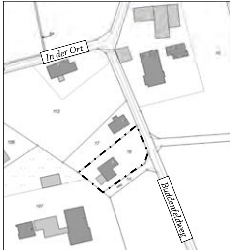
3. Änderung Bebauungsplan Nr. 18, „Südlich Bündler Straße“, Lageplan Änderungsbereich
